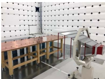
アンテナ照射試験 (ISO11452-2)
